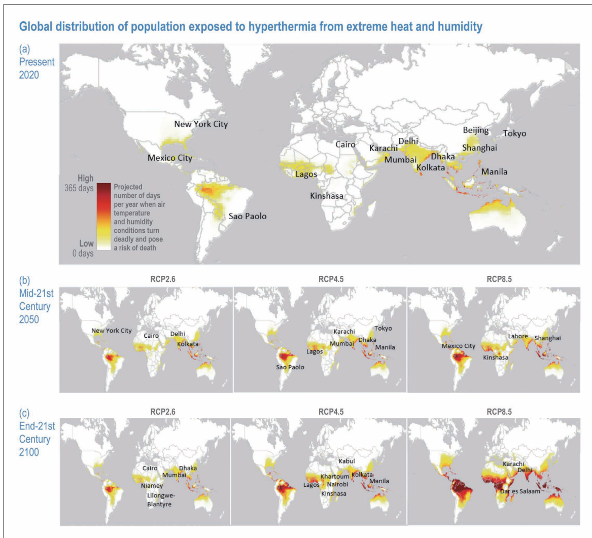
圖4.7.2.1 全球未來面對極端高溫以及高濕度的人口推估 (資料來源：IPCC WGII CH.6 Figure. 6.3)
