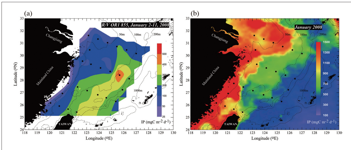
圖4.5.2.7 利用PB-E curve估算之透光層基礎生產力 (a) 與衛星測量數值分布 (b) 之比較 (兩者單位不同) (資料來源：Gong et al., 2017)
