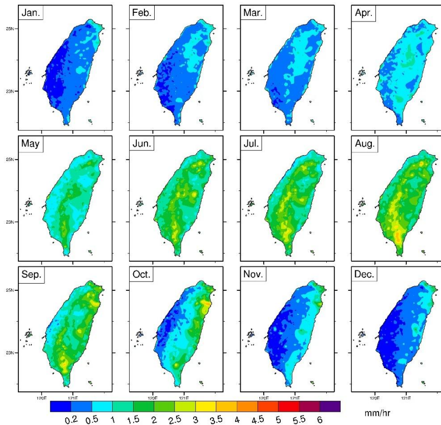
圖 4、網格化不確定性分析，進行交叉驗證實驗後的均方根誤差空間分布。(單位 mm/day)
