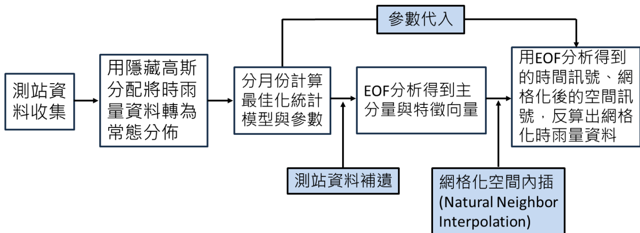
圖 1、時降雨資料產製流程
