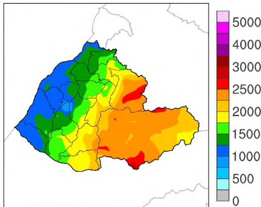
總降雨量
