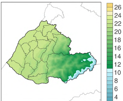
年均溫
