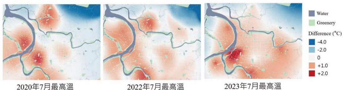
圖4.7.2.3 近年臺北 7 月都市熱島趨勢以及高溫擴張轉移分布圖
