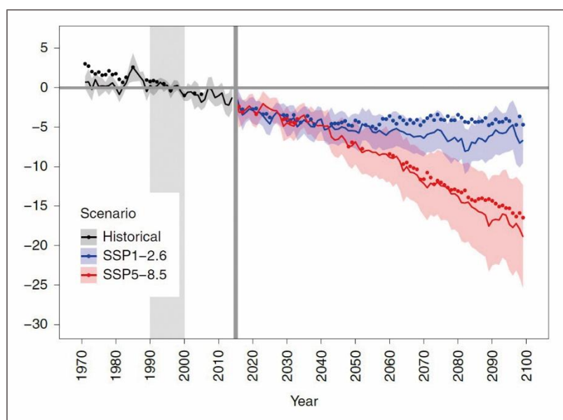
圖4.5.2.1 CMIP6預測未來全球海洋生物量的變化趨勢
