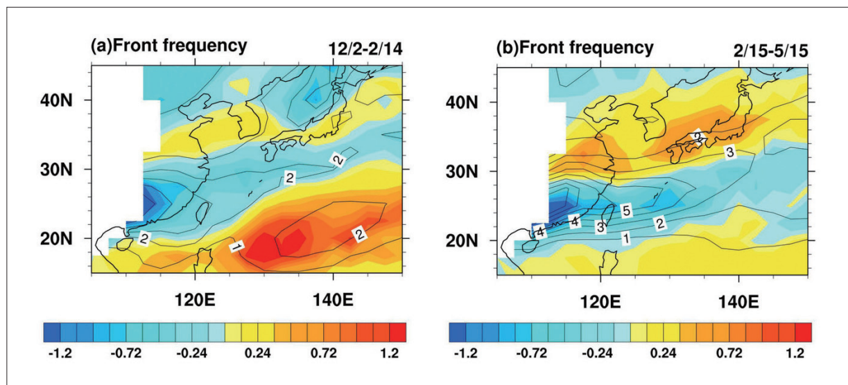
圖1.5.6 CMIP5模擬東亞地區之鋒面天數及未來變化，等值線為歷史模擬 (1976年至2005年平均；單位： \text{day season}^{-1} )，色階為RCP8.5情境於世紀末之變化量 (2071年至2100年；單位： \text{day season}^{-1} )。 (a) 冬季 (12/2至2/14)；(b) 春季 (2/15至5/15)，僅選用表現較佳的模式。(摘自 Wang et al., 2021)
