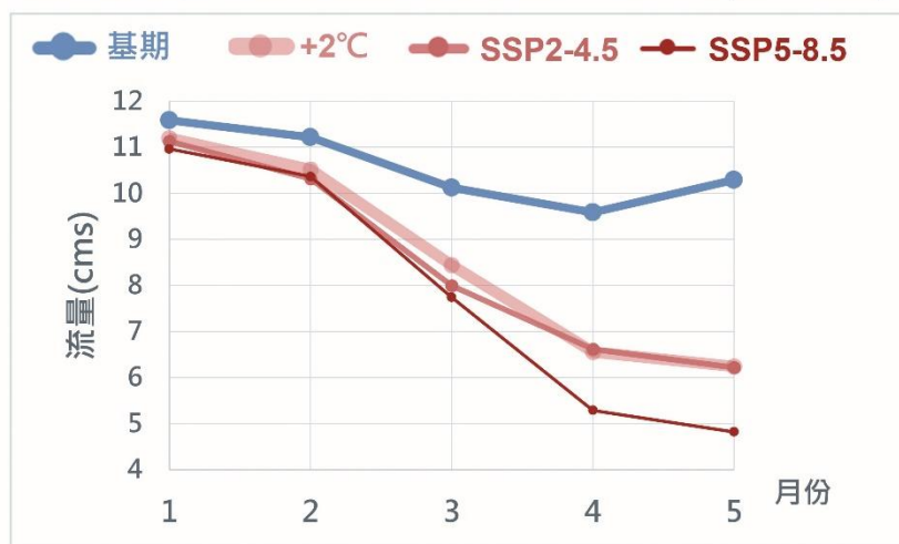
圖4.1.2.3 不同氣候變遷情境下高屏溪流域之水源潛能量 (資料來源：經濟部水利署水利規劃試驗所，2022)
