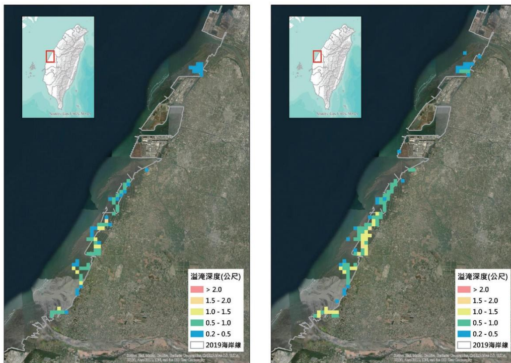
圖4.3.2.1 彰化縣海平面上升溢淹衝擊圖 (左：1.5°C情境；右：2°C情境)
