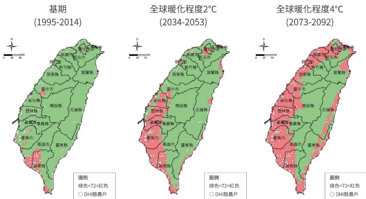
圖4.1.2.3 不同氣候變遷情境下高屏河流域之水源潛能量
