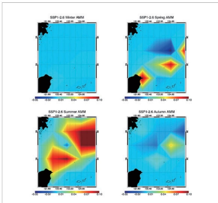
圖4.4.3.12 以SSP1-2.6 及SSP2-4.5推估2040年劍尖槍鎖管資源趨勢 (資料來源：TCCIP計畫產製)
