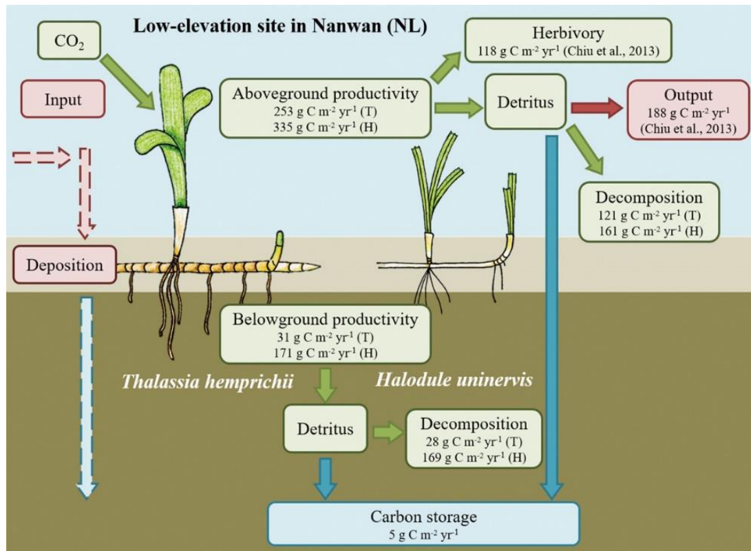
圖4.5.2.3 墾丁南灣潮間帶泰來草及單脈二藥草海草床的碳收支流程
