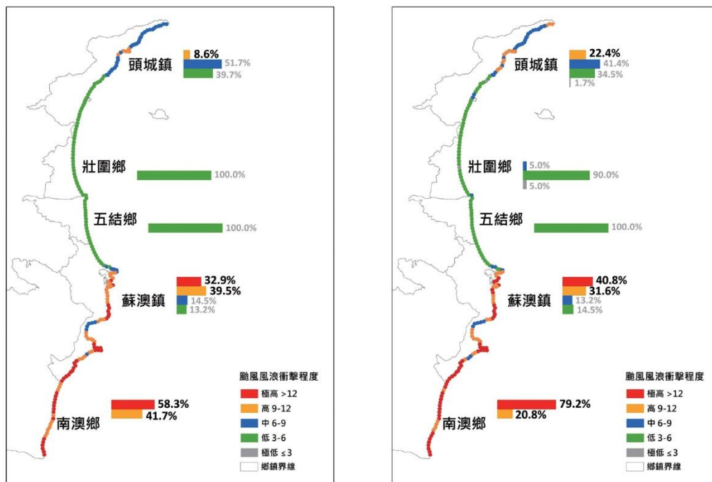
圖4.3.3.6 宜蘭縣各臨海行政區，在基期 (左圖) 與RCP8.5 (右圖) 情境下，臺灣海岸最大颱風風浪衝擊及各級距所佔該行政區海岸線百分比圖 (資料來源：TCCIP計畫產製)
