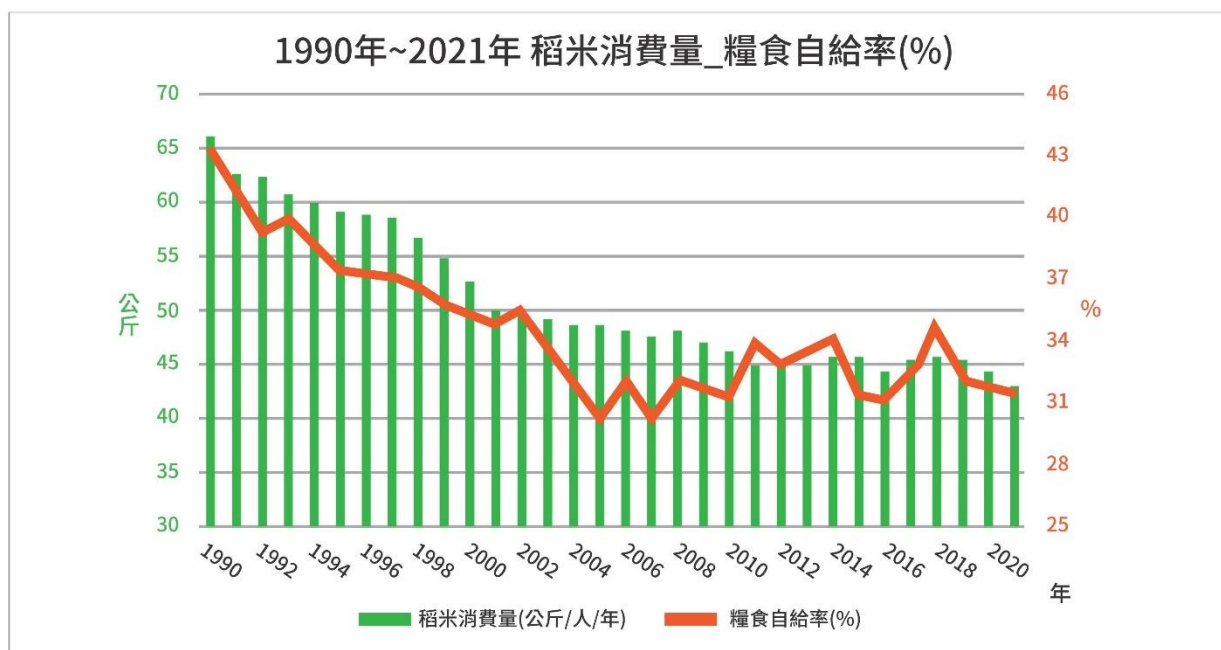
圖4.4.1.2 1990年至2021年臺灣糧食自給率及稻米食用量之變化
