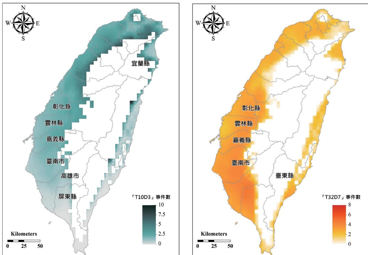
圖4.4.3.5 AR6暖化情境之低溫與高溫危害基期事件數
