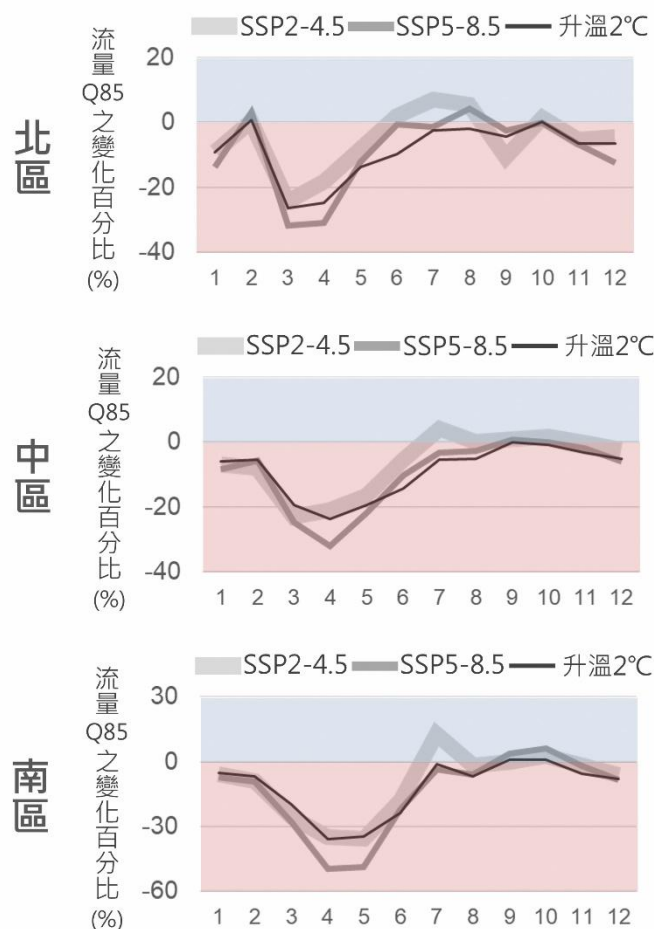
圖4.1.2.4 不同氣候變遷情境下各月份流量Q85之變化
