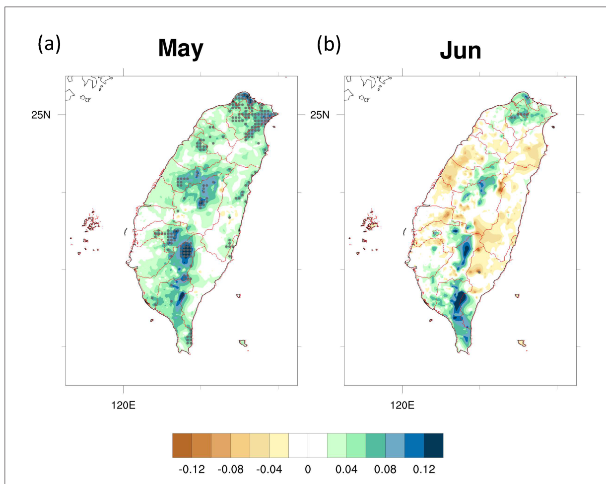
圖2.6.12 臺灣梅雨期月平均日雨量之線性趨勢 (1960年至2020年)。(a) 5月 (b) 6月，單位為 \text{mm year}^{-1} ，打點地區表示通過5%顯著性檢定。(資料來源：本報告產製)
