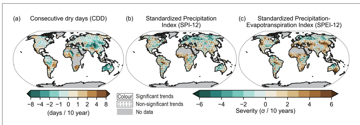
圖1.4.7 (a) 1960年至2018年之 (年) 最長連續不降雨日 (Maximum number of consecutive dry days, CDD) 的線性趨勢；(b) 1951年至2016年之12個月SPI 和 (c) 12個月SPEI 的觀察線性趨勢。灰色代表缺乏足夠數據的區域，x區域表示統計趨勢不顯著。因此，無重疊的顏色區域表示趨勢具有統計顯著性。(摘自IPCC AR6, WGI, Figure 11.17)
