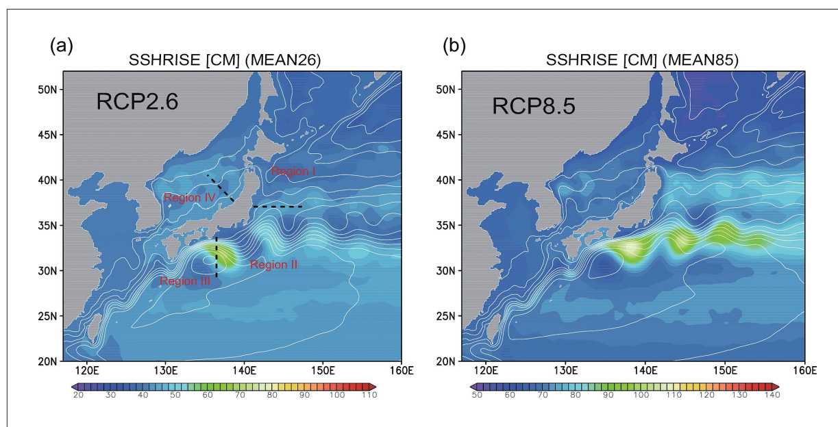
圖1.3.12 CMIP5 (a) RCP2.6與 (b) RCP8.5暖化情境下區域降尺度海洋模擬的海平面高度上升分布 (2081年至2100年平均與1986年至2005年歷史模擬平均之差異)。(摘自Yamanaka et al., 2020)
