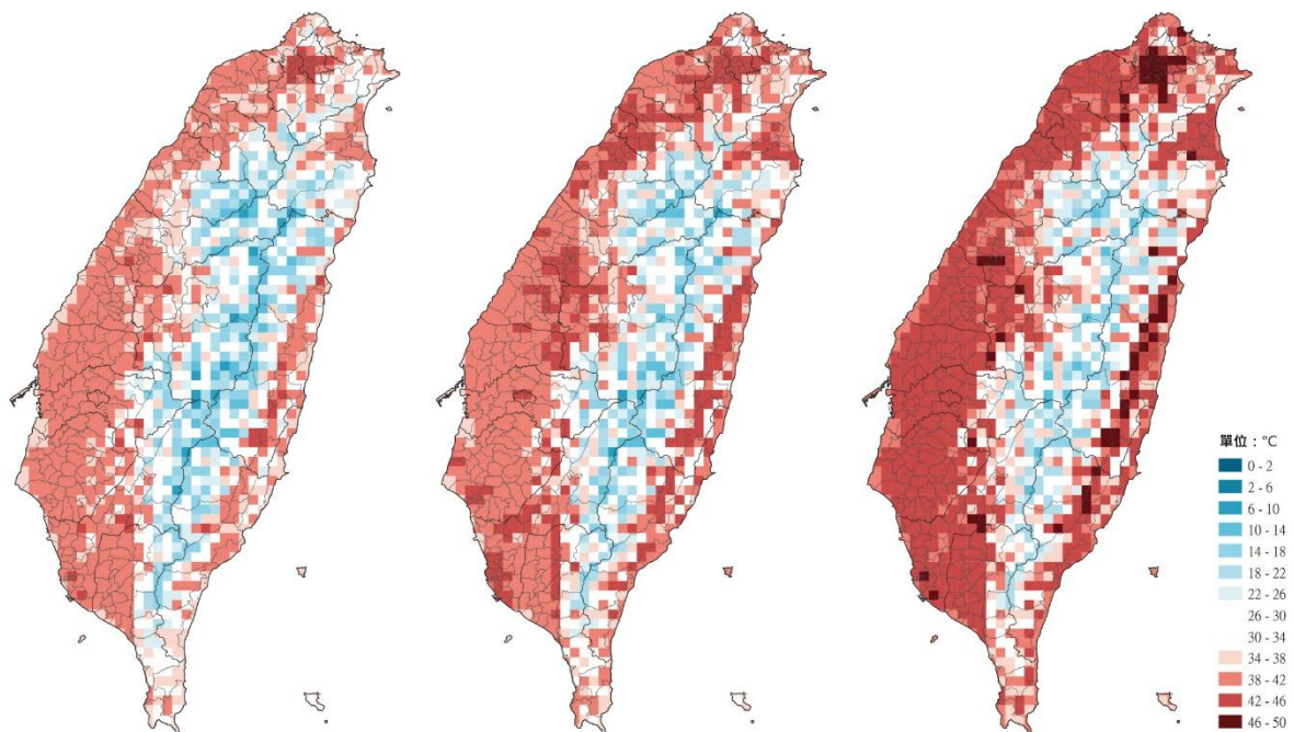
圖4.7.2.4 全臺生理等效溫度 (PET) 分布圖
