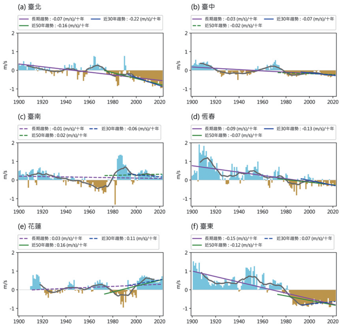
圖2.4.1 1900年至2022年6個百年署屬測站年平均風速的距平值時間序列圖。測站分別是 (a) 臺北、(b) 臺中、(c) 臺南、(d) 恆春、(e) 花蓮與 (f) 臺東測站。橫軸為年份，1900年至2022年，縱軸為相對於各測站氣候值 (1961年至1990年) 的風速距平，正距平為藍色柱狀，負距平為咖啡色柱狀，曲線為15年滑動平均值。近30年、近50年及長期 (1900年至2022年) 趨勢線分別以藍、綠及紫色表示，實線表示趨勢值通過5%顯著性檢定，虛線則未通過。(資料來源：中央氣象署，本報告產製)
