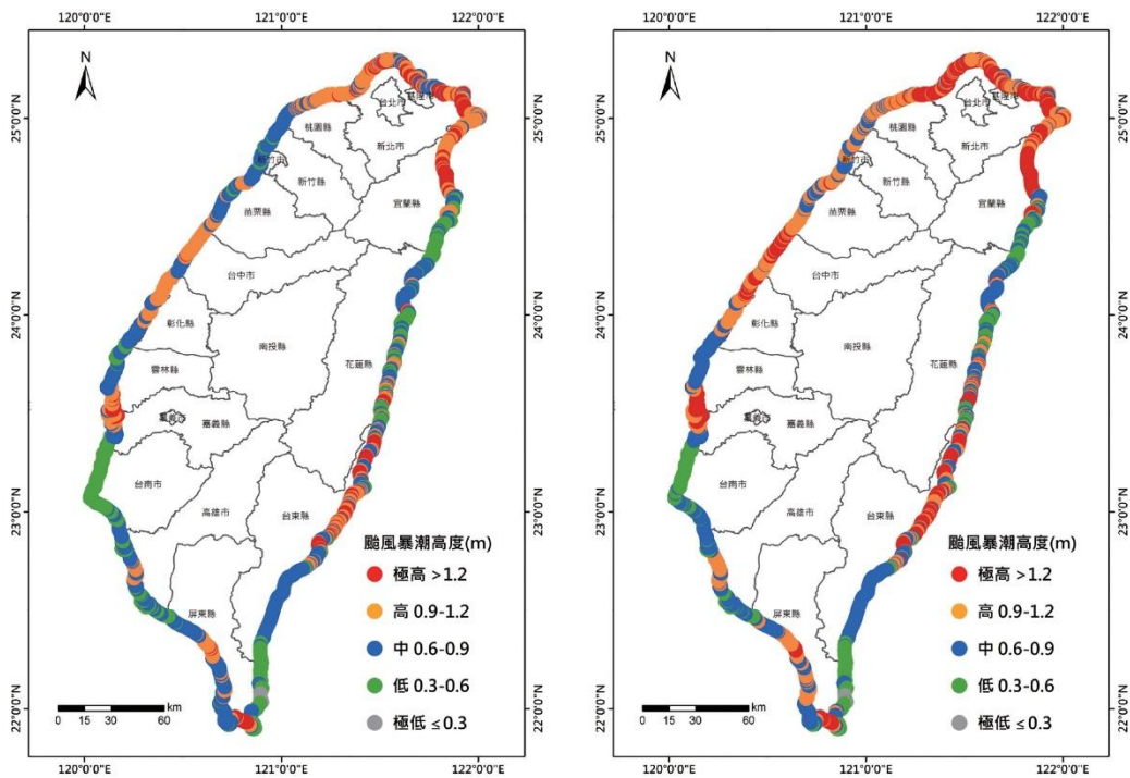
圖4.3.3.3 臺灣海岸最大颱風暴潮偏差衝擊圖 (左圖基期情境；右圖RCP8.5情境) (資料來源：TCCIP計畫產製)
