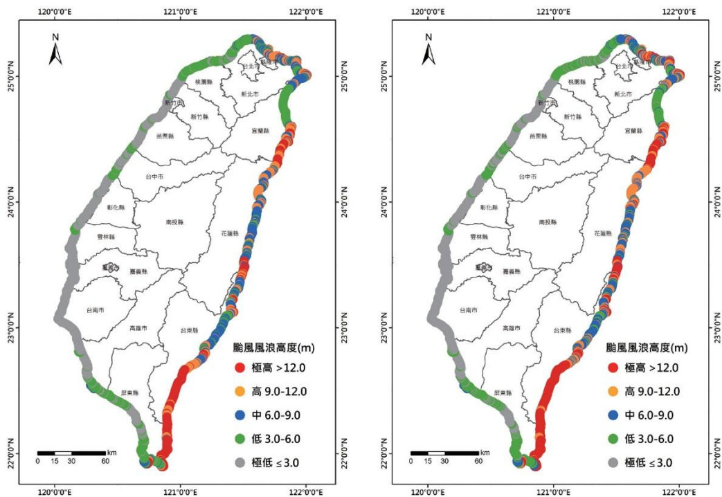
圖4.3.3.4 臺灣海岸最大颱風風浪衝擊圖 (左圖基期情境；右圖RCP8.5情境) (資料來源：TCCIP計畫產製)
