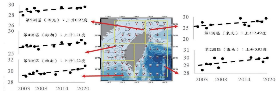
圖4.4.3.11 2003年至2020年臺灣周邊海域夏季海面水溫分析調查 (a) 四季不同水深 (5m、25m)之空間變動趨勢 (b)以夏季為例之分區變動趨勢 (資料來源：嚴國維等人，2021)
