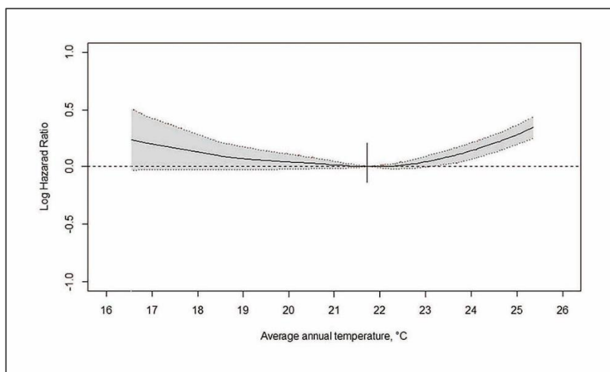
圖4.6.2.3 溫度與重鬱症發病率的反應曲線長期暴露於溫度和重鬱症發病率的劑量 - 反應曲線。註：實線表示對數風險比，灰色區域表示95%信賴區間。(資料來源：Chen et al., 2019)
