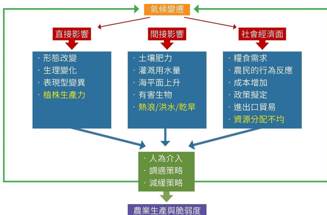
圖4.4.1.1 氣候變遷對農業生產的直接、間接和社會經濟影響
