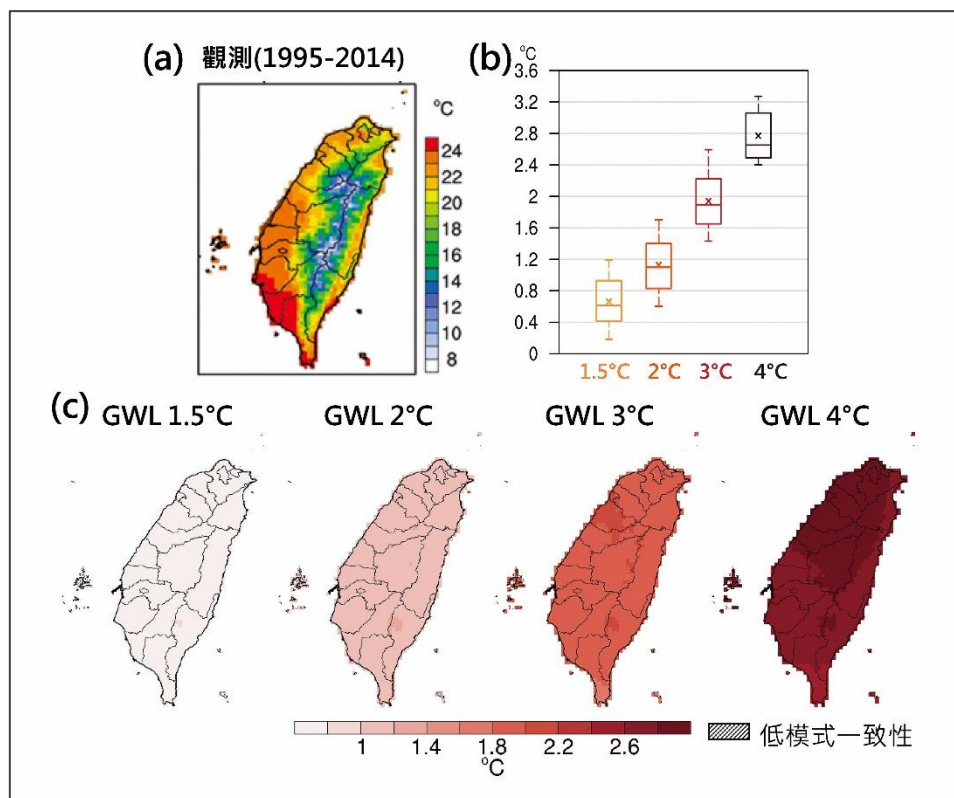
圖3.2.3 歷史與GWL下臺灣平均溫度變化。 其中歷史氣候使用TCCIP網格化觀測，未來推估則為統計降尺度資料。(a) 圖為基期 (1995年至2014年) 觀測氣候年平均溫度分佈 (單位：°C)；(b) 圖為GWL 1.5°C、GWL 2°C、GWL 3°C、GWL 4°C相對於模式現今氣候 (1995年至2014年)，以盒鬚圖第95、75、50、25、5百分位數 (由上至下) 呈現模式氣候平均溫度變化分佈範圍 (單位：°C)，X記號為系集平均值。(c) 圖為GWL溫度變化 (模式中位數) 空間分布 (單位：°C)，斜線區域為低模式一致性。GWL下各模式或各情境的詳細時間區間可參考臺灣氣候變遷關鍵指標圖集：AR6統計降尺度版 (2023)。(資料來源：本報告產製)
